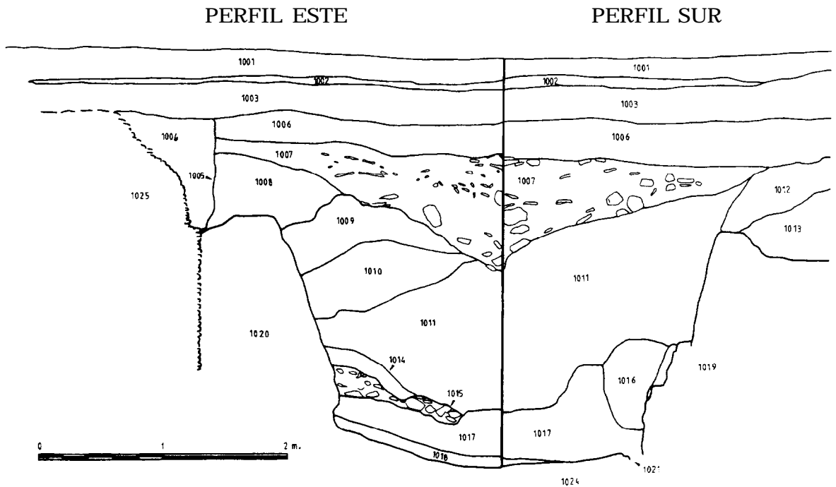
FIGURA 5: Estratigrafía del Sondeo I
