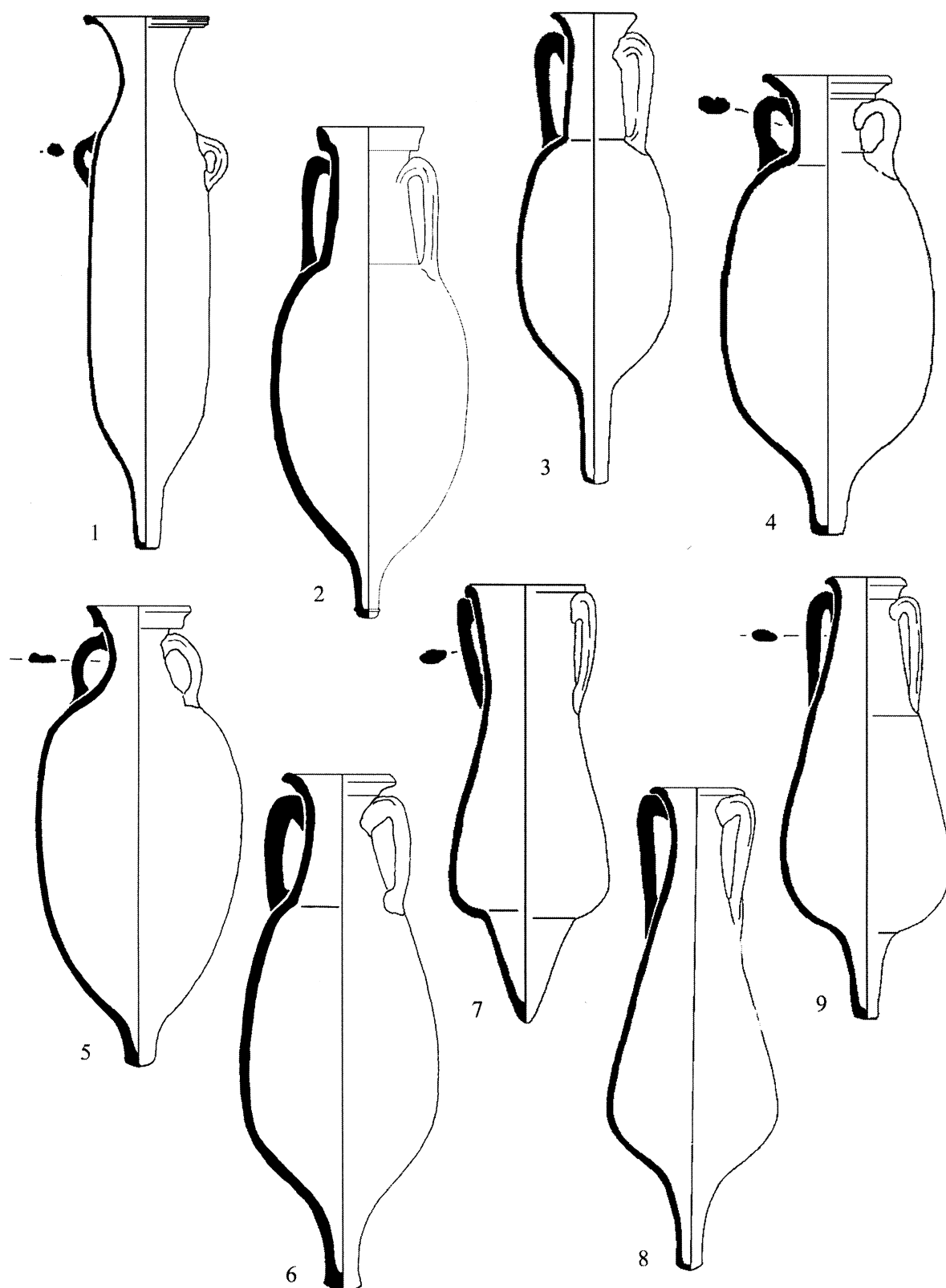
Figura 1.- Ánforas salsarias altoimperiales béticas. 1.- Mañá C2; 2.- Dressel 7; 3.- Dressel 8; 4.- Dressel 9; 5.- Dressel 10; 6.- Dressel 11; 7.- Beltrán IIA; 8.- Beltrán IIB; 9.- Pompéi VII.
